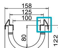
VISTA FRONTALE
